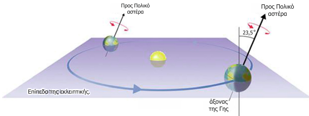
Εικόνα 4: Γραφική αναπαράσταση επιπέδου της τροχιάς της ετήσιας περιφοράς της Γης γύρω από τον Ήλιο. Ο άξονας ημερήσιας περιστροφής της Γης σχηματίζει γωνία 23.5° με τον άξονα περιφοράς.
